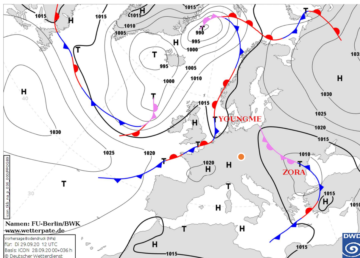
Weather Chart, TUE, 29.09.2020, 14:00 CEST
