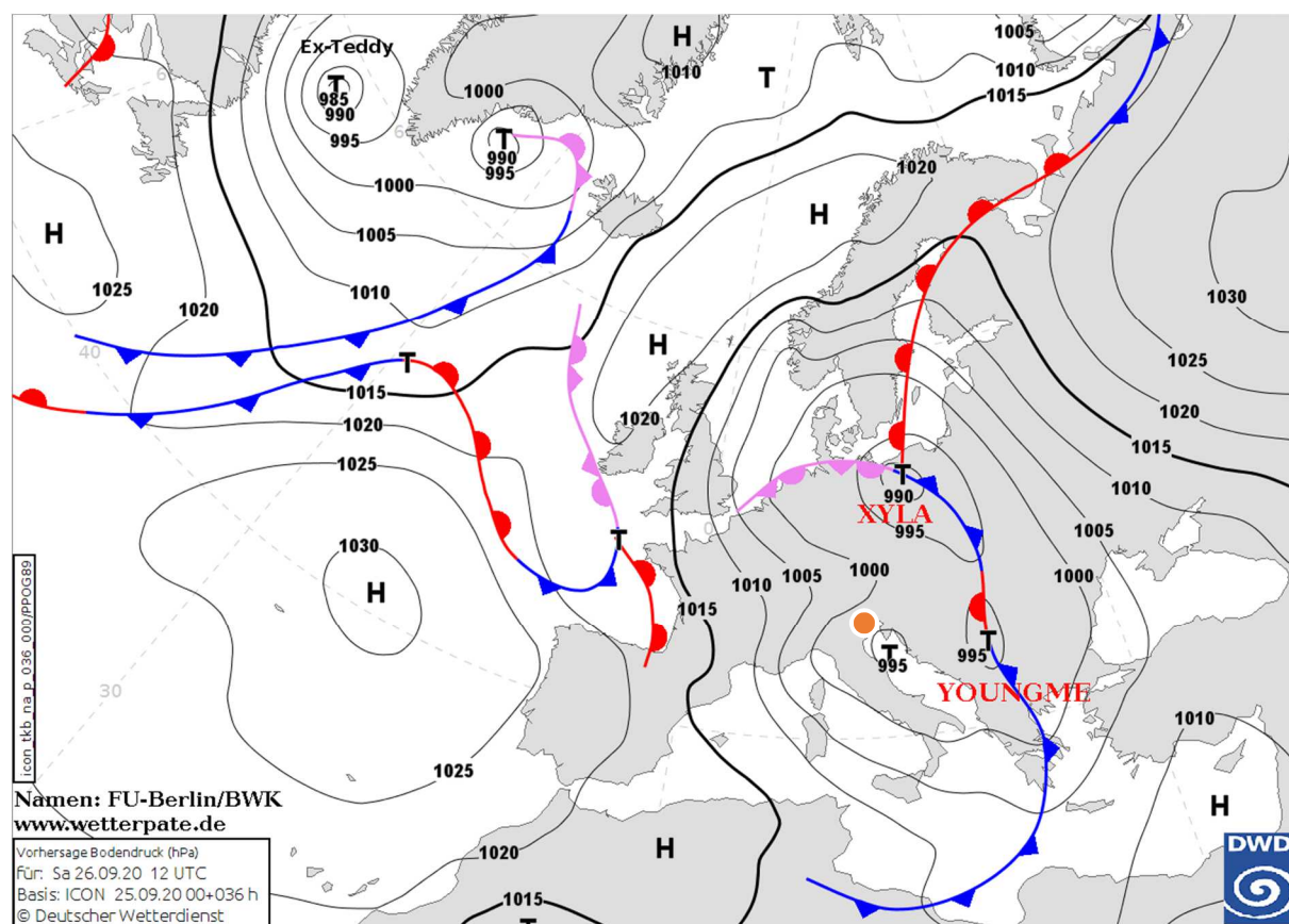
Weather Chart, SAT, 26.09.2020, 14:00 CEST
